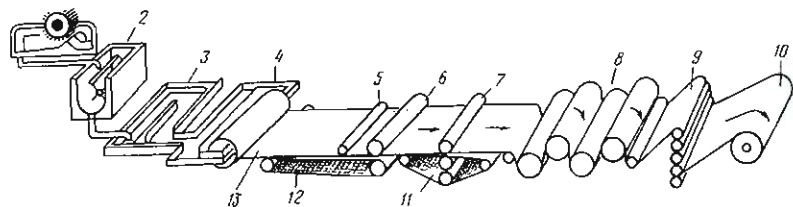
Схема производства бумаги (по Граллерту и Грушке): 1 – ролл (размол); 2 – мешальный чан; 3 – песочница; 4 – узлоловитель; 5 – ровнитель с водяными знаками; 6 – гаучпресс; 7 – мокрый пресс; 8 – сушильная часть; 9 – лощильная часть; 10 – станина наката; 11 – бесконечное сукно; 12 – бесконечное сито; 13 – бумажное полотно
